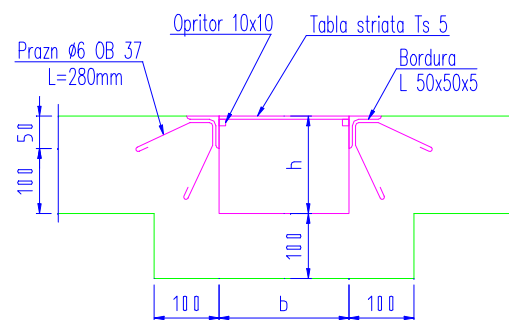
Sc. 1:10
